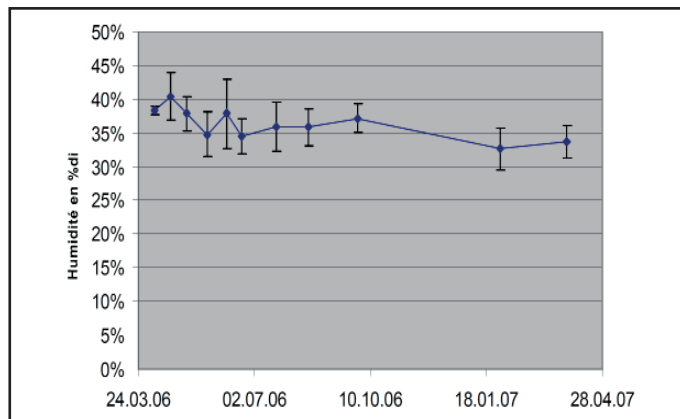
Processus de séchage du bois d'épicéa à l'état non déchiqueté
