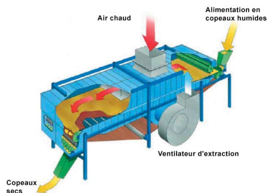
Principe du séchoir à bande (W. Kunz dryTec AG. 2005).
