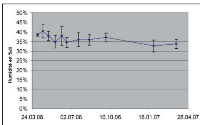
Processus de séchage du bois de hêtre à l'état non déchiqueté (Elber, 2007).
