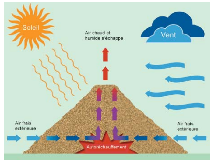
Principe du séchage par convection naturelle (LWF, 2014).
