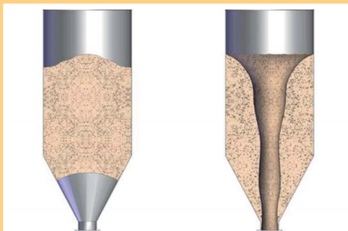
Formation de ponts (à g.) et de puits (à d.) (Hinterreiter, 2010).
